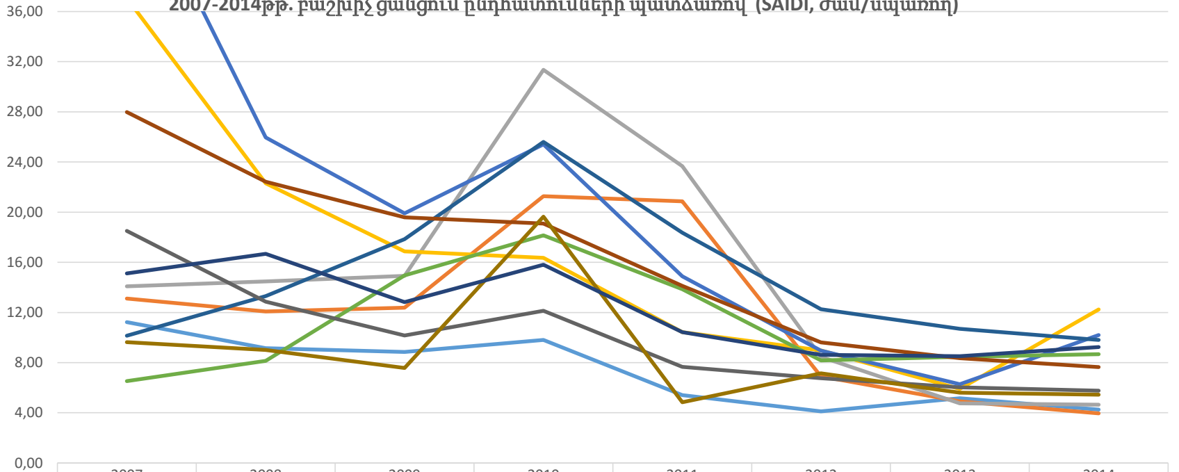
Մեկ սպառողին բաժին ընկնող էլեկտրամատակարարման ընդհատումների միջին տարեկան տևողությունը Հայաստանի Հանրապետության մարզերում և Երևան քաղաքում 2007-2014թթ. բաշխիչ ցանցում ընդհատումների պատճառով (SAIDI, ժամ/սպառող)
