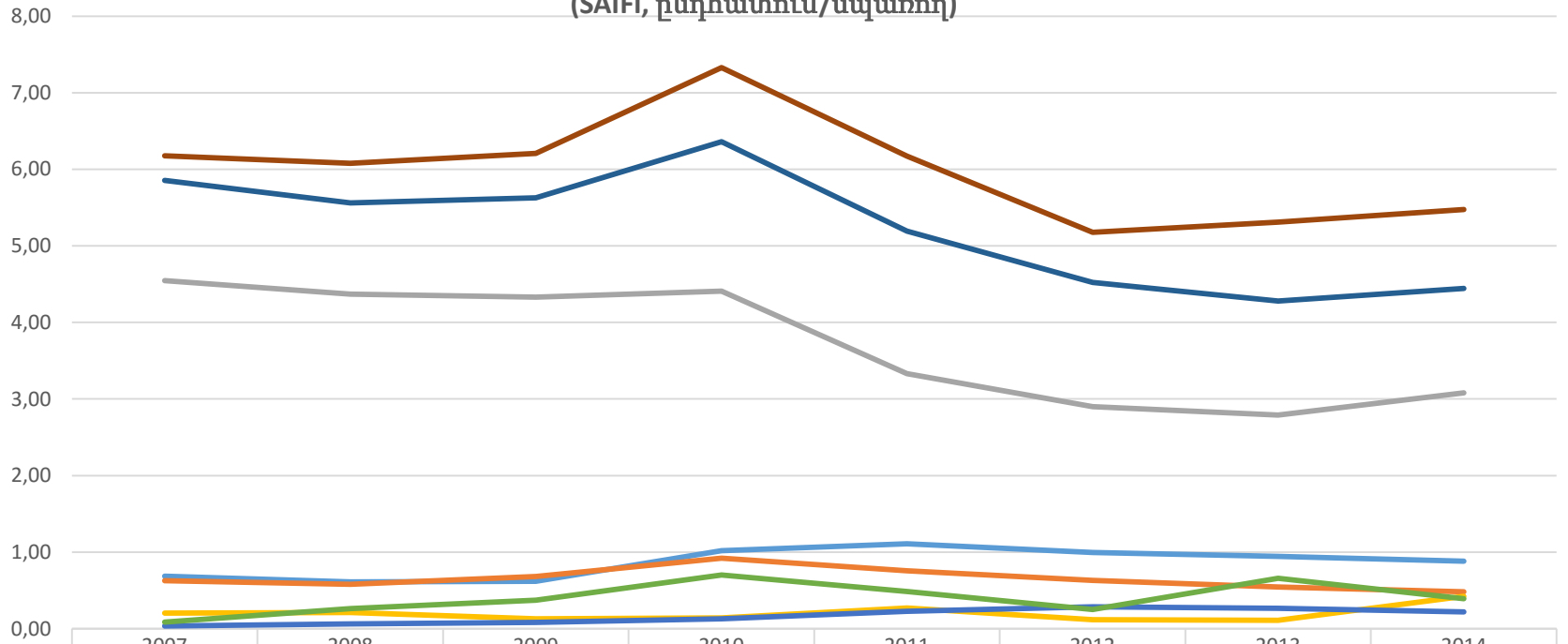
Մեկ սպառողին բաժին ընկնող էլեկտրամատակարարման ընդհատումների միջին տարեկան քանակությունը Հայաստանի Հանրապետությունում 2007-2014թթ. (SAIFI, ընդհատում/սպառող)
