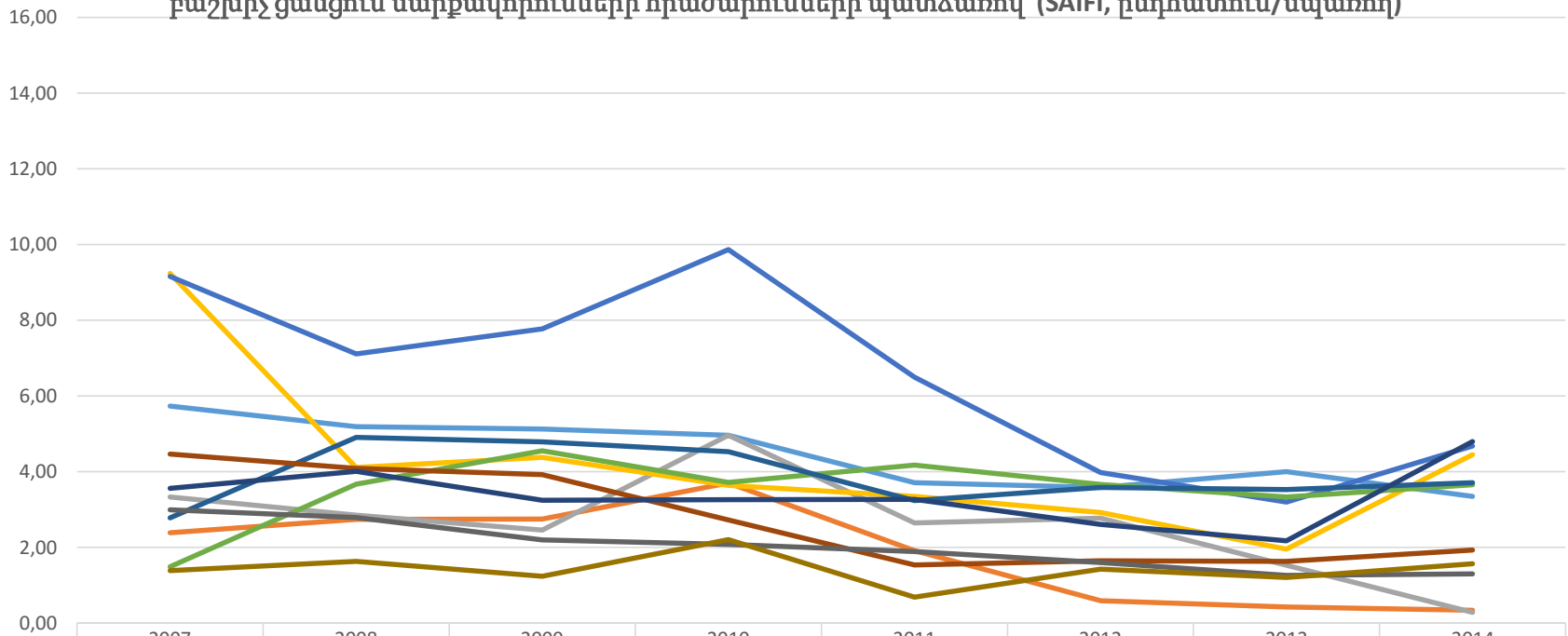
Մեկ սպառողին բաժին ընկնող էլեկտրամատակարարման ընդհատումների միջին տարեկան քանակությունը Հայաստանի Հանրապետությունում 2007-2014թթ. բաշխիչ ցանցում սարքավորումների հրաժարումների պատճառով (SAIFI, ընդհատում/սպառող)
