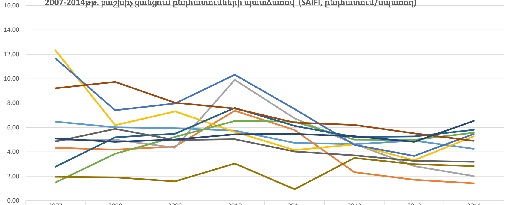
Մեկ սպառողին բաժին ընկնող էլեկտրամատակարարման ընդհատումների միջին տարեկան քանակությունը Հայաստանի Հանրապետության մարզերում և Երևան քաղաքում 2007-2014թթ. բաշխիչ ցանցում ընդհատումների պատճառով (SAIFI, ընդհատում/սպառող)
