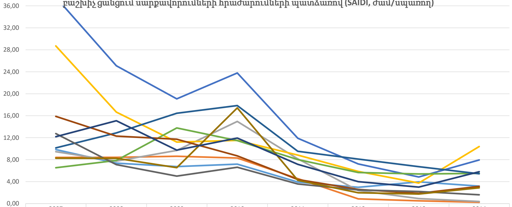
Մեկ սպառողին բաժին ընկնող էլեկտրամատակարարման ընդհատումների միջին տարեկան տևողությունը Հայաստանի Հանրապետությունում 2007-2014թթ. բաշխիչ ցանցում սարքավորումների հրաժարումների պատճառով (SAIDI, ժամ/սպառող)
