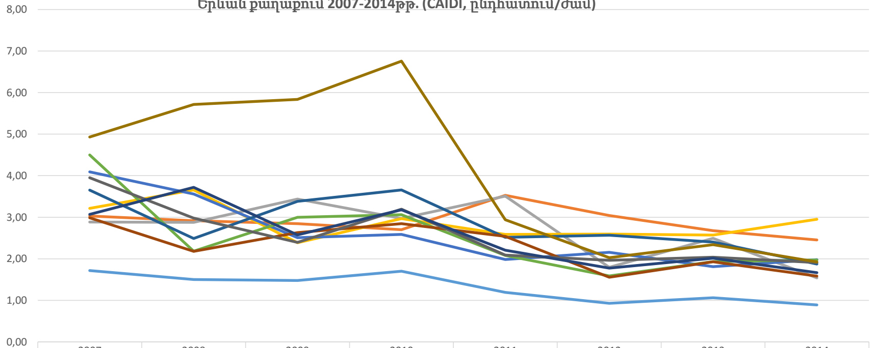
Էլեկտրամատակարարման ընդհատումների վերականգնման միջին տարեկան տևողությունը Հայաստանի Հանրապետության մարզերում և Երևան քաղաքում 2007-2014թթ. (CAIDI, ընդհատում/ժամ)
