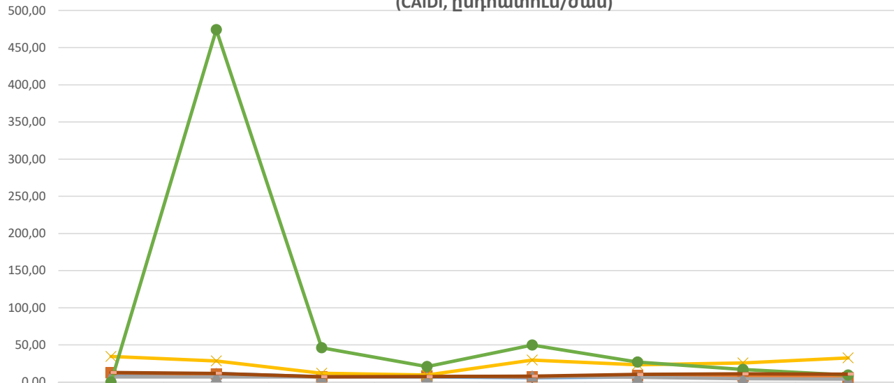
Գազամատակարարման ընդհատումների վերականգնման միջին տարեկան տևողությունը Հայաստանի Հանրապետության մարզերում 2009-2016թթ. (CAIDI, ընդհատում/ժամ)
