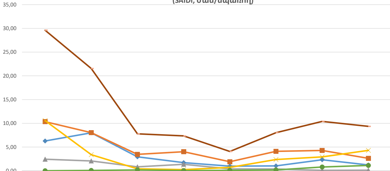
Մեկ սպառողին բաժին ընկնող գազամատակարարման ընդհատումների միջին տարեկան տևողությունը Հայաստանի Հանրապետության մարզերում 2009-2016թթ. (SAIDI, ժամ/սպառող)
