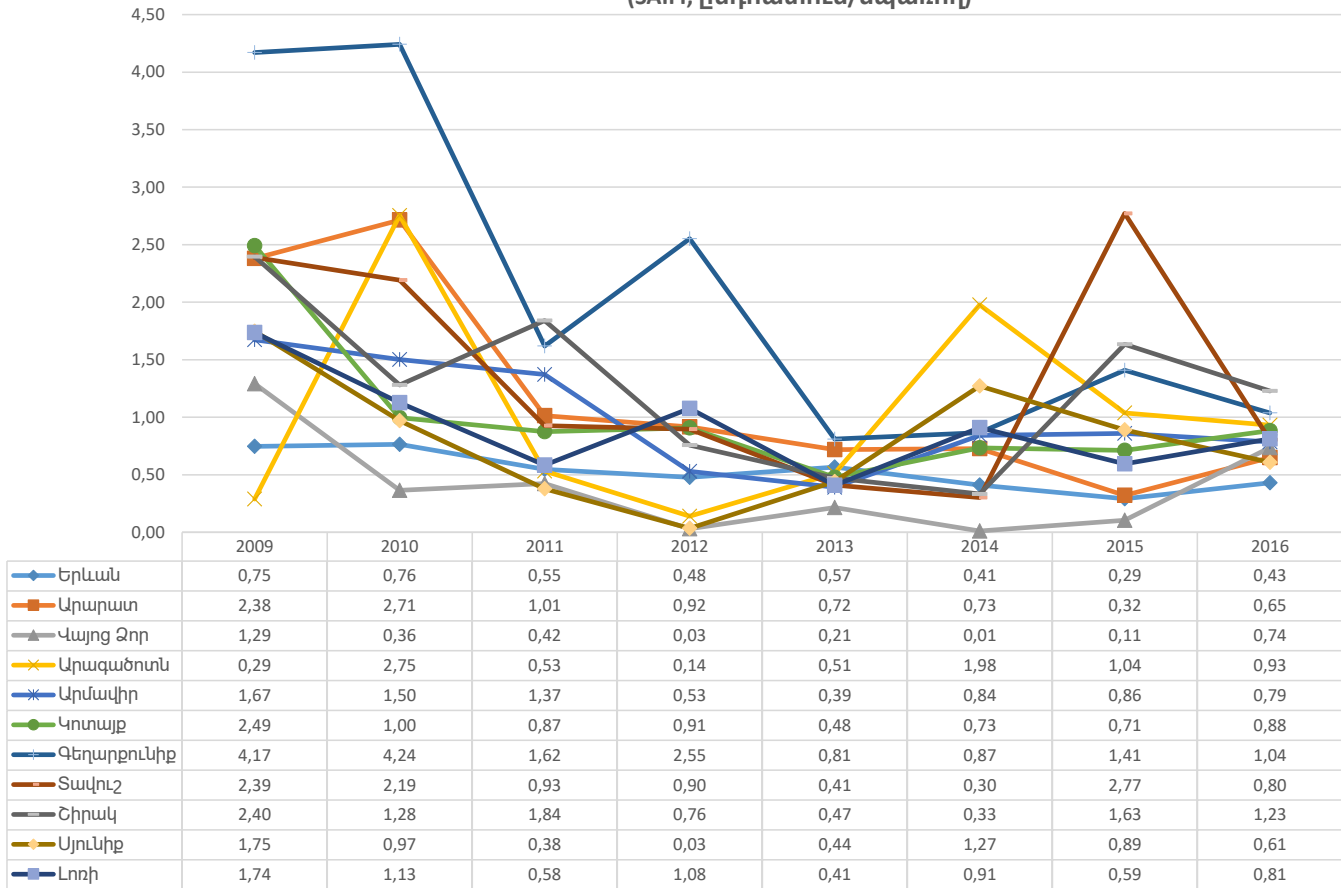
Մեկ սպառողին բաժին ընկնող զագամատակարարման ընդհատումների միջին տարեկան քանակությունը Հայաստանի Հանրապետությունում 2009-2016թթ. (SAIFI, ընդհատում/սպառող)
