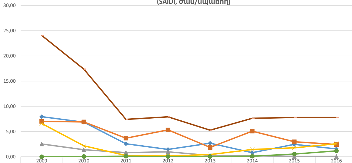
Մեկ սպառողին բաժին ընկնող գազամատակարարման ընդհատումների միջին տարեկան տևողությունը Հայաստանի Հանրապետությունում 2009-2016թթ. (SAIDI, ժամ/սպառող)
