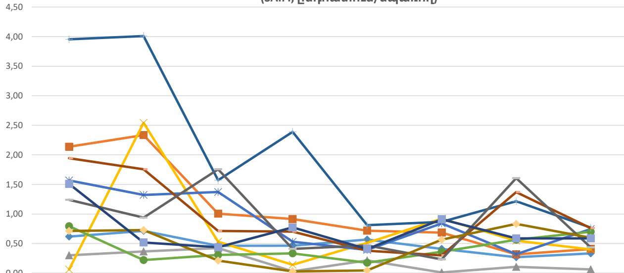
Մեկ սպառողին բաժին ընկնող զագամատակարարման ընդհատումների միջին տարեկան քանակությունը Հայաստանի Հանրապետությունում 2009-2016թթ. (SAIFI, ընդհատում/սպառող)
