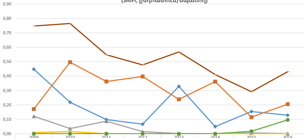
Մեկ սպառողին բաժին ընկնող գազամատակարարման ընդհատումների միջին տարեկան քանակությունը Երևան քաղաքում 2009-2016թթ. (SAIFI, ընդհատում/սպառող)
