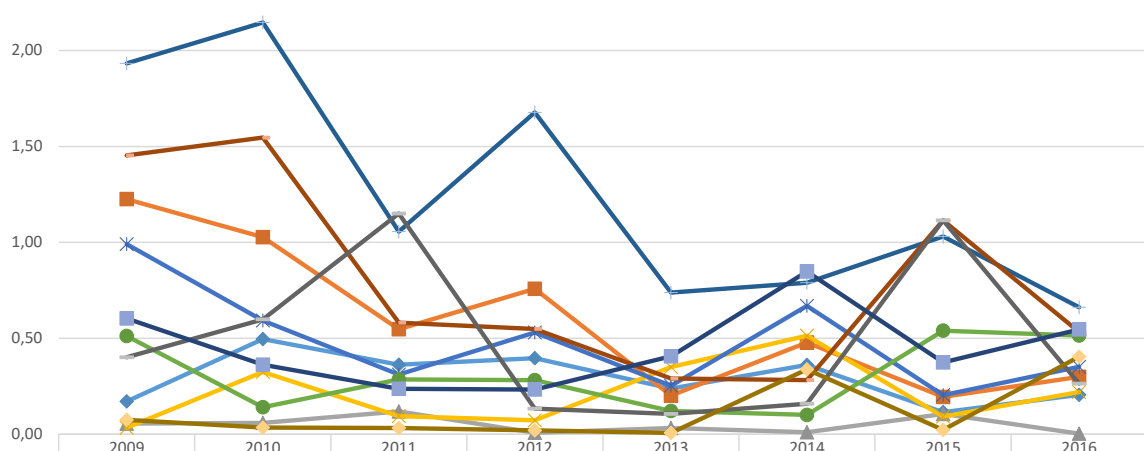
Հայաստանի Հանրապետությունում գազամատակարարման ցանցում վթարների պատճառով տեղի ունեցած մեկ սպառողին բաժին ընկնող գազամատակարարման ընդհատումների միջին տարեկան քանակությունը 2009-2016 թվականների ընթացքում (SAIFI, ընդհատում/սպառող)
