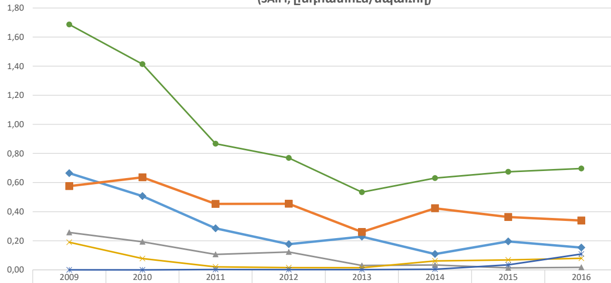
Մեկ սպառողին բաժին ընկնող զագամատակարարման ընդհատումների միջին տարեկան քանակությունը Հայաստանի Հանրապետությունում 2009-2016թթ. (SAIFI, ընդհատում/սպառող)
